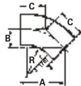
45° Horizontal Bend
